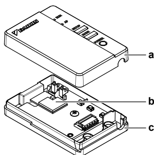
a Górna obudowa b Płytki drukowane adaptera sieci bezprzewodowej LAN
