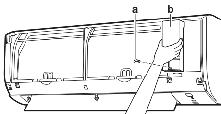
a Śruba pokrywy serwisowej
