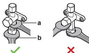
a Klucz maszynowy b Klucz dynamometryczny
