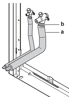
a Materiał izolacyjny b Uszczelnienie itp.
