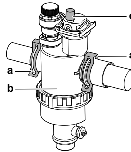
a Zacisk b Filtr magnetyczny/separator zanieczyszczeń c Zawór odpowietrzający
