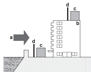
a Wiatr nadmorski b Budynek c Urządzenie zewnętrzne d Wiatrochron
