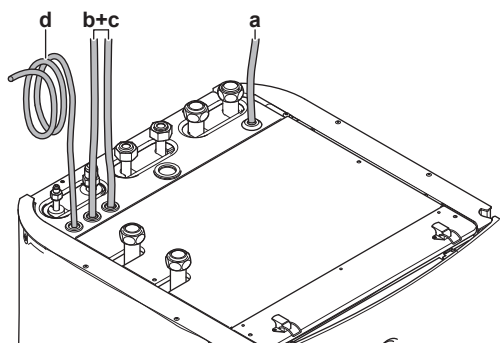
a, b, c Okablowanie w miejscu instalacji (patrz tabela poniżej) d Zamontowany fabrycznie przewód zasilania grzałki BUH
