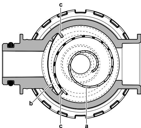
a Filtr zwinięty b Filtr siatkowy c Wypustka
