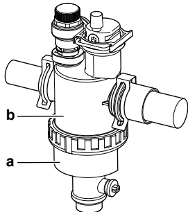
a Odkręcana część dolna b Obudowa filtra wody
