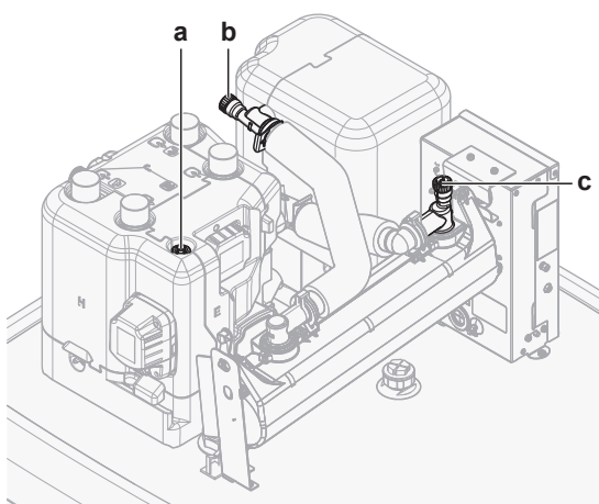
a, b, c Ręczny zawór odpowietrzający
