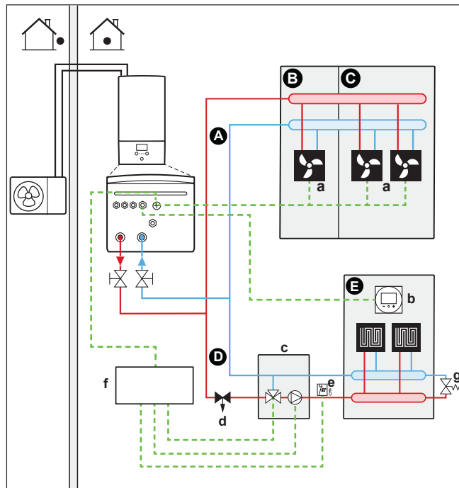
2 System z separatorem hydraulicznym dla strefy głównej:
