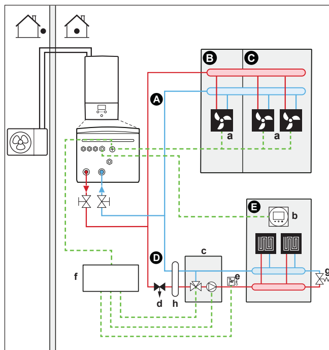
3 System z separatorem hydraulicznym dla obu stref:
