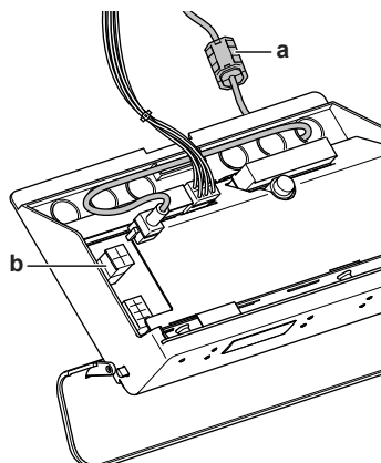
a Cewka elektromagnesu b Złącze X5
