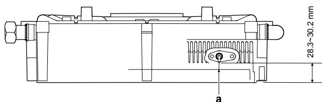
a Przerwa iskry (±4,5 mm)
