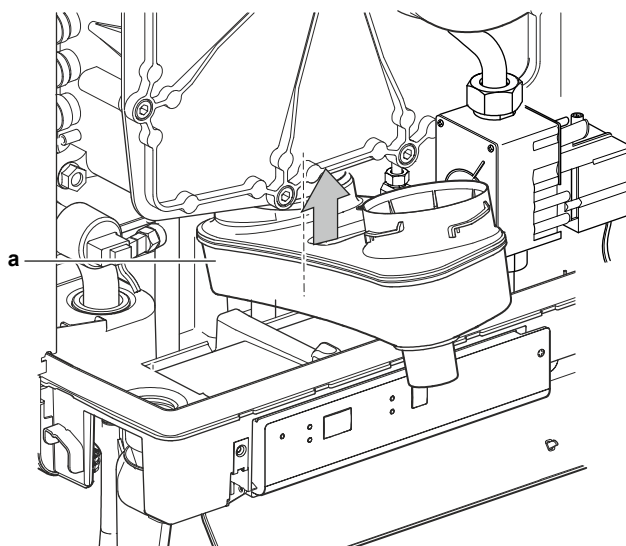
a Taca podstawowa
