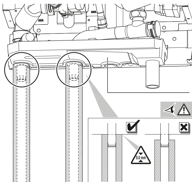
a Zestaw tacy na skropliny
