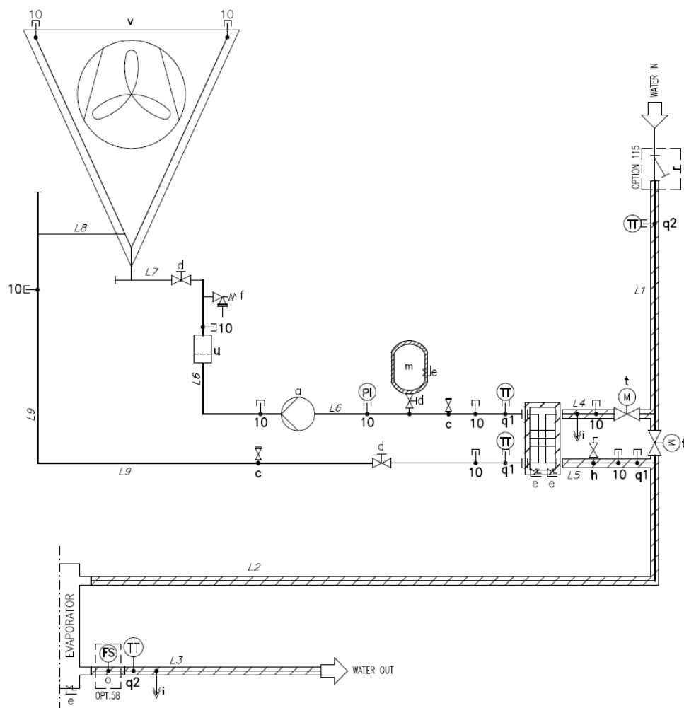
Rys. 21– Zamknięta pętla Hydronic Bezpłatne chłodzenie P&ID (op. 231)
