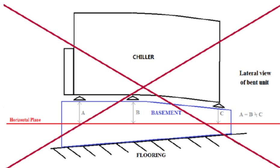
Rys. 13– Pозиomowanie jednostki
