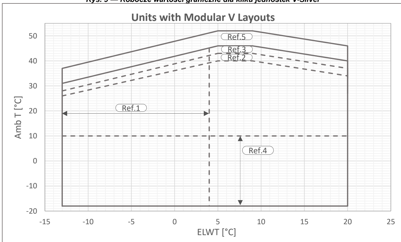
Rys. 10 — Robocze wartości graniczne dla kilku jednostek V-Gold
