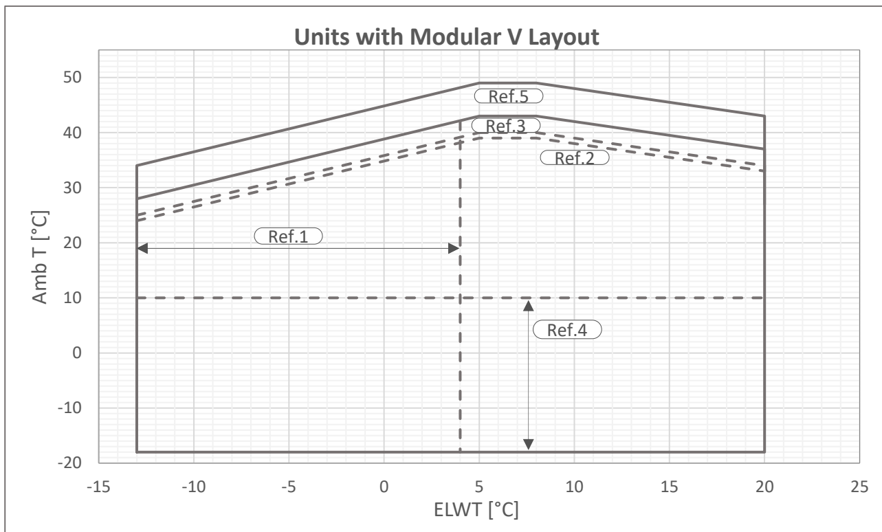
Rys. 9 — Robocze wartości graniczne dla kilku jednostek V-Silver
