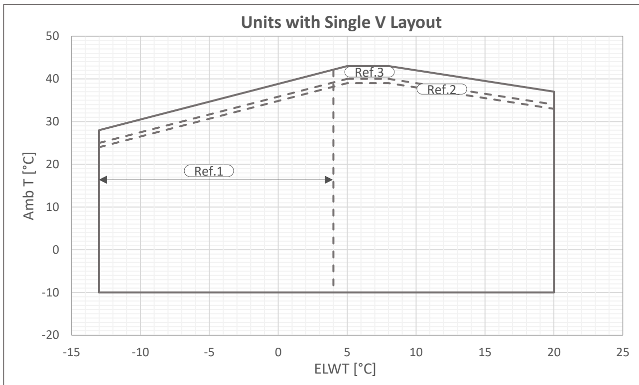
Rys. 11 — Robocze wartości graniczne dla pojedynczej jednostki V-Silver
