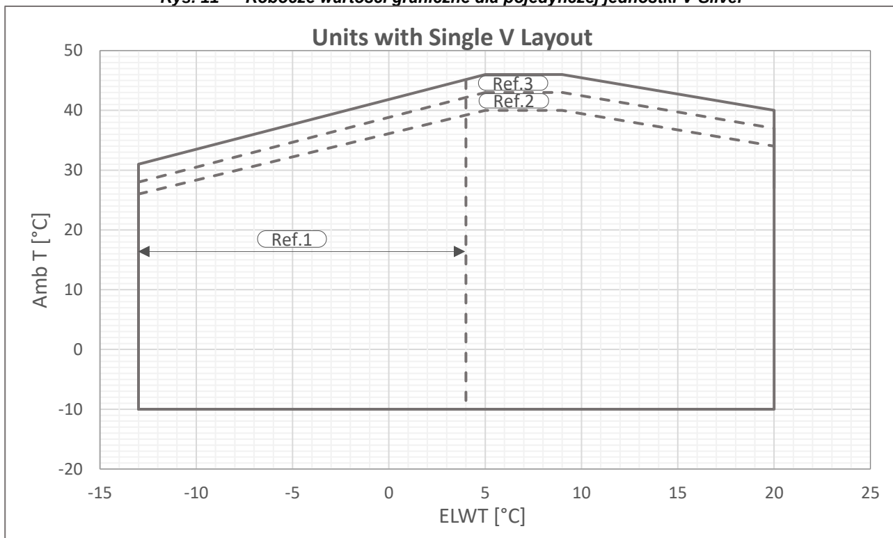
Rys. 12 — Robocze wartości graniczne dla pojedynczej jednostki V-Gold
