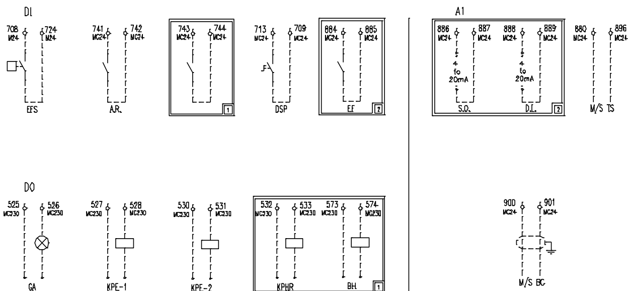
Rysunek 8 – Połączenia elektryczne jednostki w miejscu instalacji
