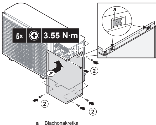
a Blachonakrętka
