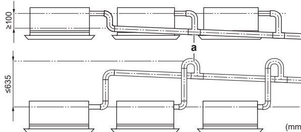
a Trójnik T
