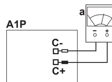
A1P Główna płytko drukowana a Multimetr C Punkty pomiaru napięcia resztkowego
