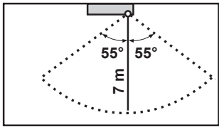
Kąt w płaszczyźnie poziomej (z góry)
