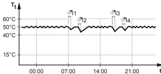
T_t Temperatura zbiornika buforowego t Godzina
